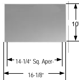
16" Sq. 70W—175W
